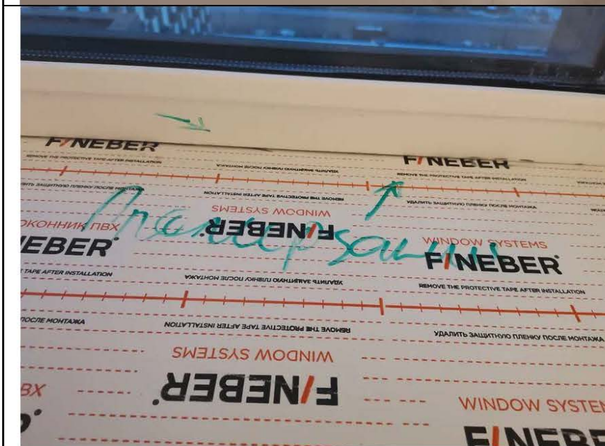
Фото №51. Дефекты профиля ПВХ и щели в оконном блоке на кухне квартиры.
